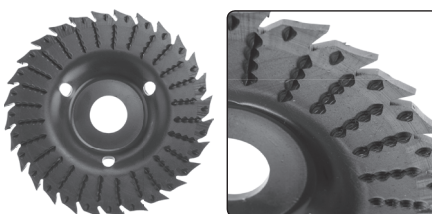
Obr. 10, Rašpľové kotúče
